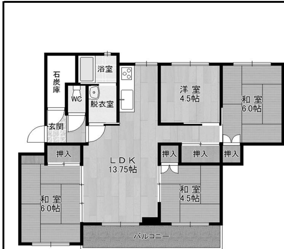
間取り図（大家族世帯向け）
